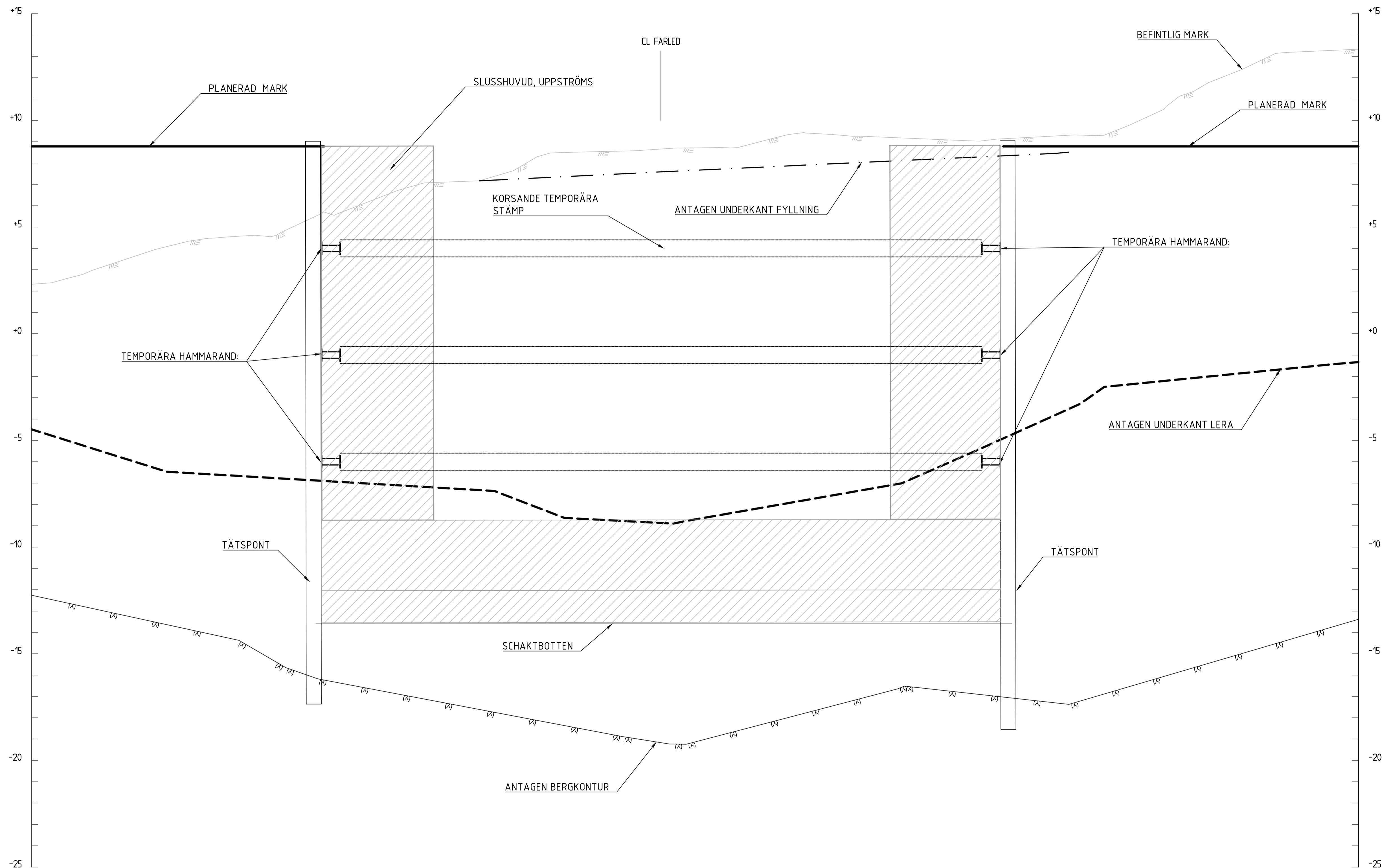
SEKTION C-C (1/020, S.14+TK.T.A00-BDC.R.101) 1:100
